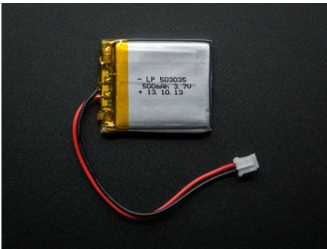
Lithium Ion Polymer Battery - 3.7v 500mAh ( http://adafru.it/1578 )
